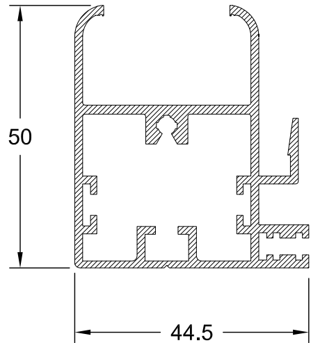
353 - ΟΡΙΖ. PROFIL ΜΕ ΓΑΝΤΖΟ 1.085 gr/m
