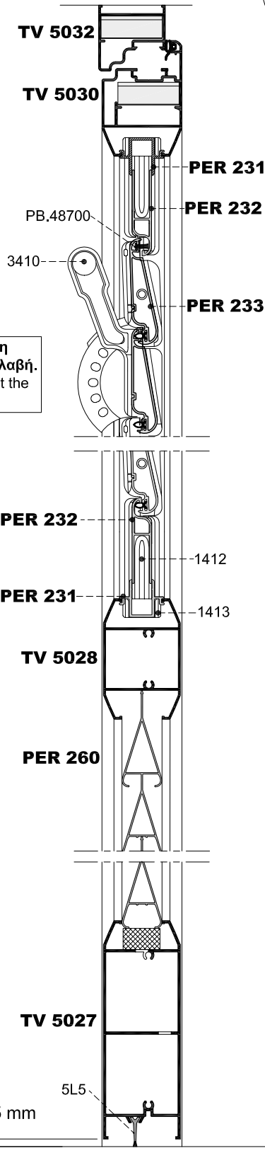
Μηχανισμός κινητής περσίδας TEKNALSYSTEM Mechanism of movable fixed louver TEKNALSYSTEM
