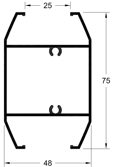
ΧΩΡΙΣΜΑ ΠΑΤΖΟΥΡΙΟΥ TRANSOM / MULLION FOR SHUTTER
