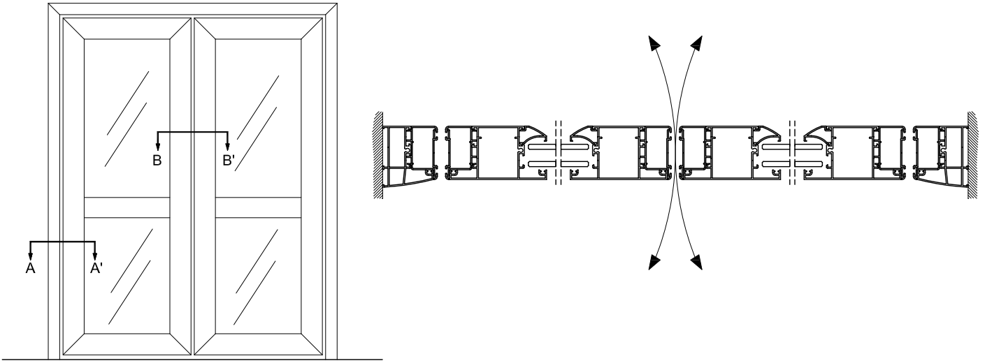
TOMH A-A' SECTION A-A'
