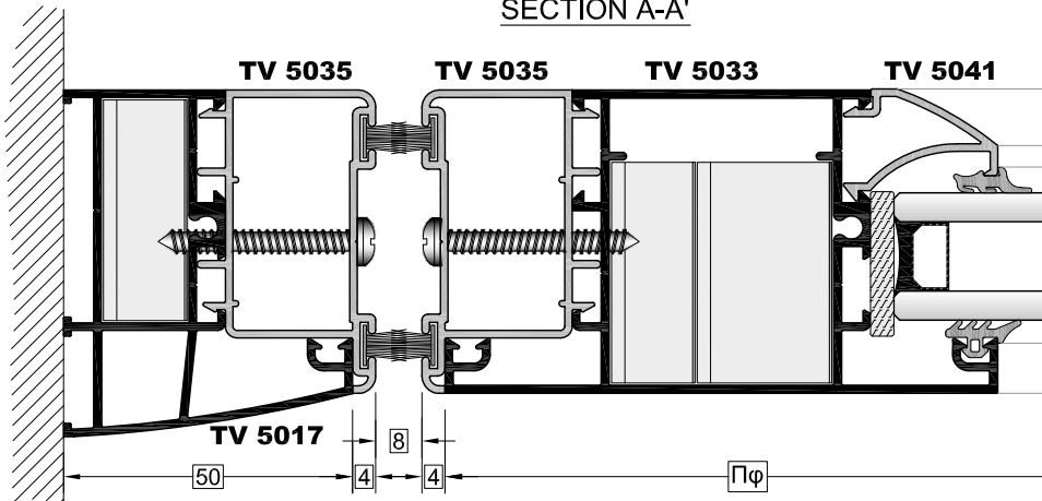
TOMH A-A' SECTION A-A'
