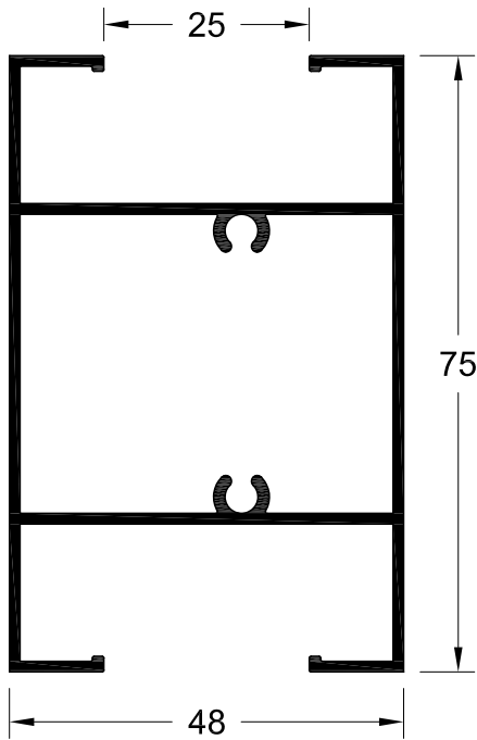
ΙΣΙΟ ΧΩΡΙΣΜΑ ΠΑΤΖΟΥΡΙΟΥ STRAIGHT TRANSOM / MULLION PROFILE
