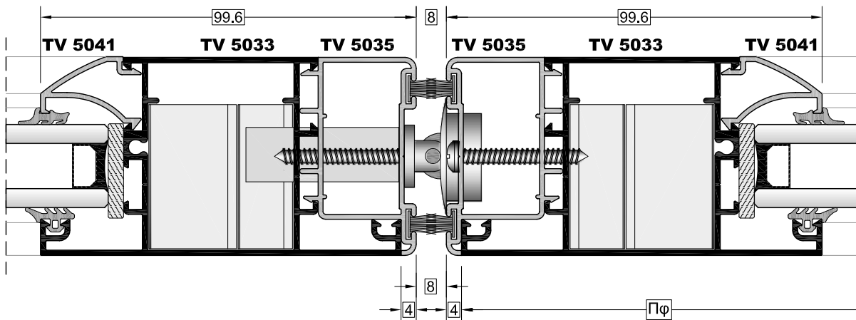
TOMH B-B' SECTION B-B'
