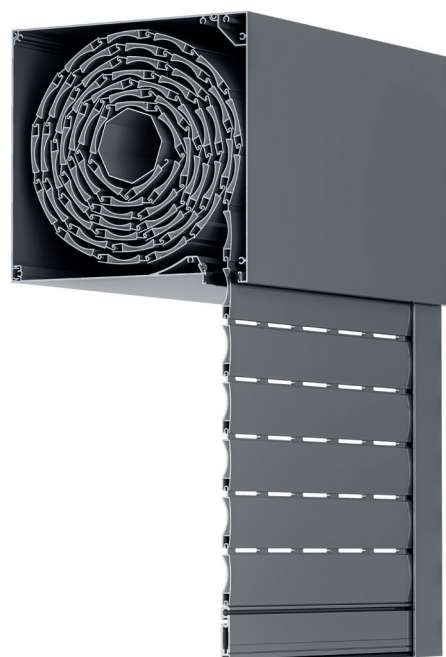
Τομή κουτιού συστήματος ERS 960 Section of ERS 960 System Box
